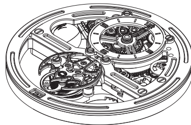
BM05机心
